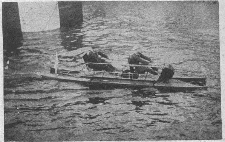
Expériences d'Hydroglisseurs sur la Seine. — Différents hydroglisseurs ont été expérimentés. Notre photo montre un des modèles.
